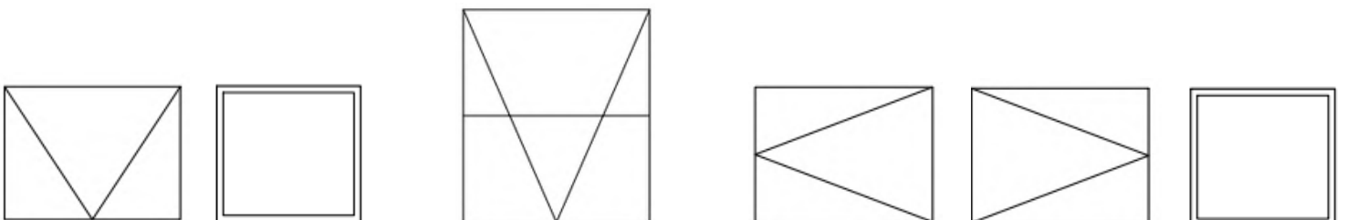
HEIGHT: 380 mm / WIDTH: 400;450;500; 600; 700;800;900;1000 mm
